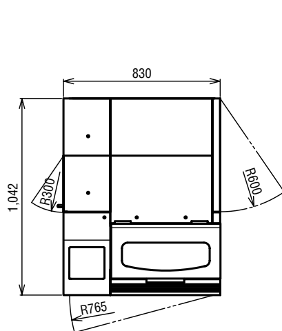
平面図
