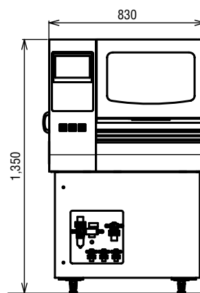
正面図
