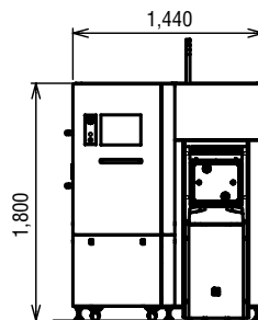
正面図
