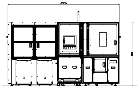
正面図
