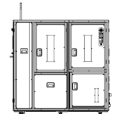
右側面図
