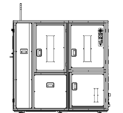
右側面図
