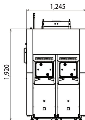
正面图
