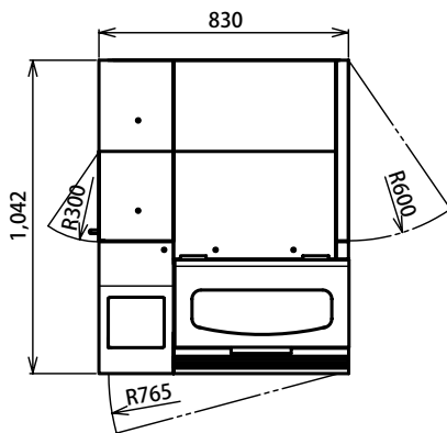
平面图
