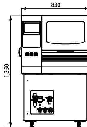
正面图
