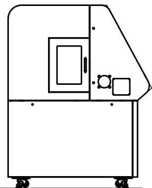
左侧面图
