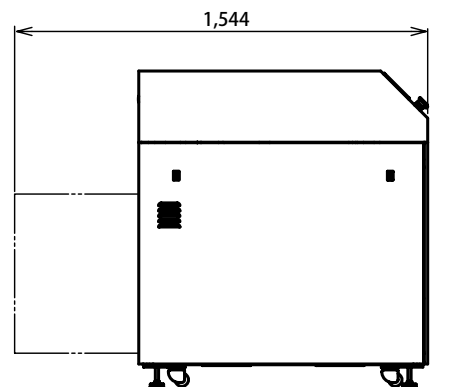
左侧面图
