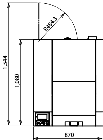
平面图
