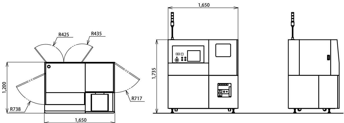
平面图
